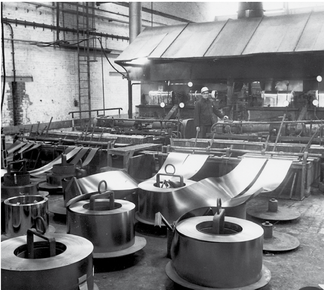
Inbetriebnahme der ersten elektolytischen Bandverzinnungsanlage der Welt (1934), Andernach
